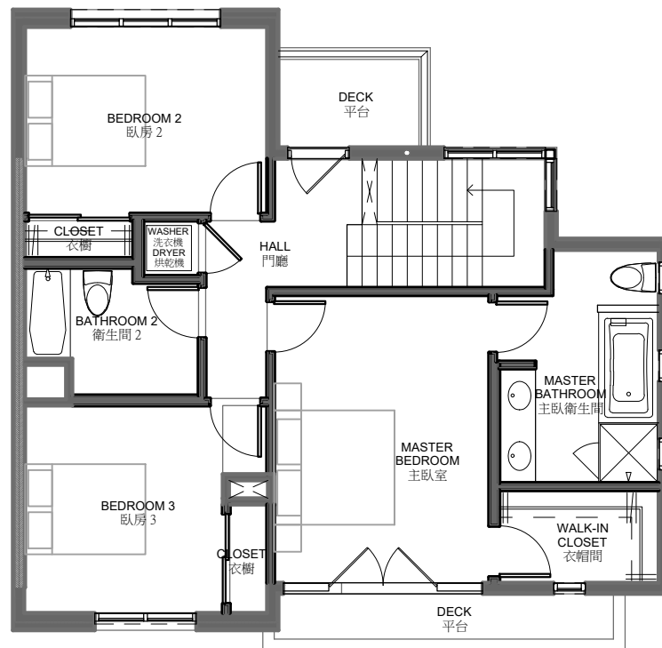
Second Floor Plan 1,007 S.F. 二樓平面圖
