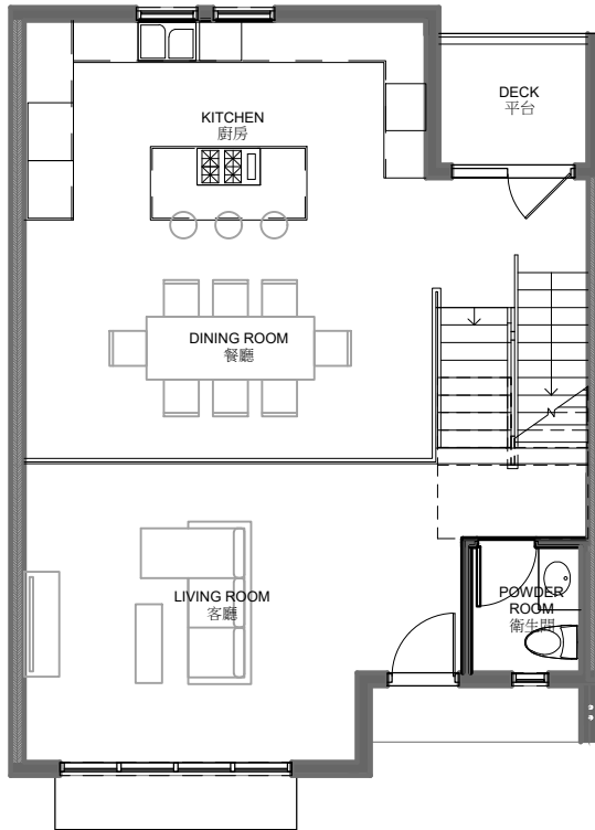
First Floor Plan 935 S.F. 一樓平面圖
