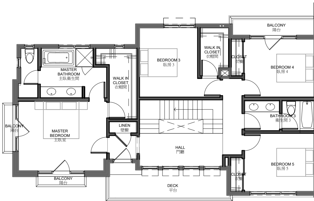
Second Floor Plan 1,338 S.F. 二樓平面圖
