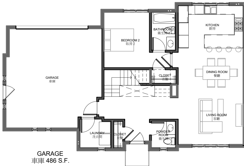
First Floor Plan 1,005 S.F. 一樓平面圖
