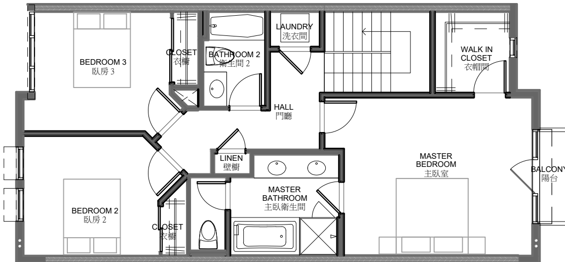
Second Floor Plan 1,000 S.F. 二樓平面圖
