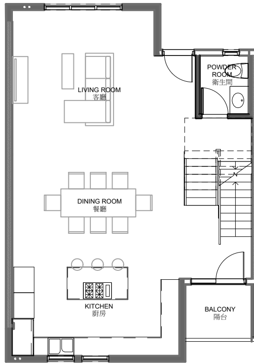
First Floor Plan 919 S.F. 一樓平面圖
