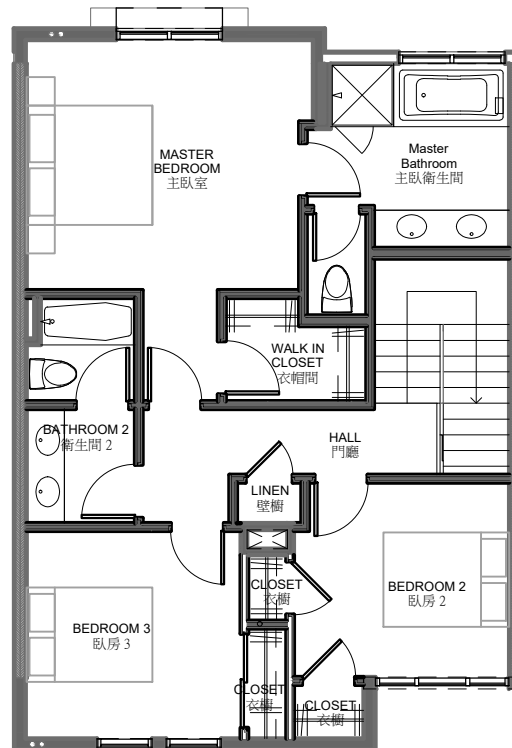
Second Floor Plan 967 S.F. 二樓平面圖
