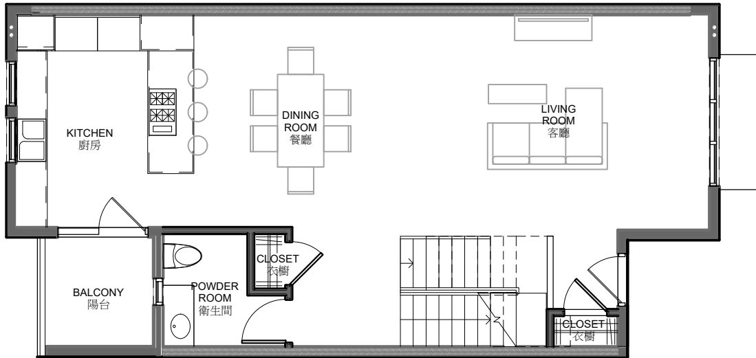
First Floor Plan 875 S.F. 一樓平面圖
