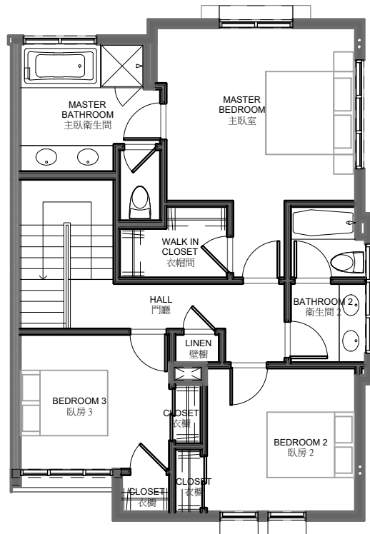
Second Floor Plan 988 S.F. 二樓平面圖
