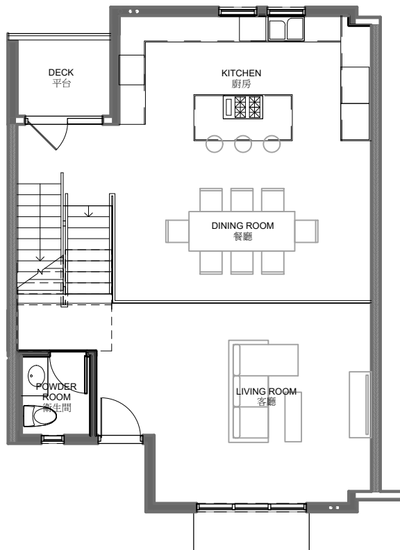
First Floor Plan 967 S.F. 一樓平面圖
