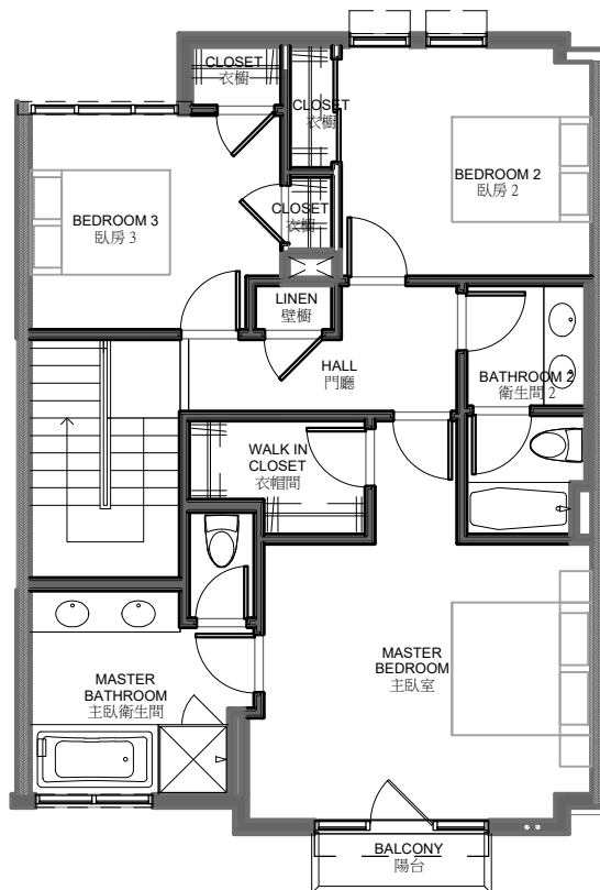
Second Floor Plan 1,011 S.F. 二樓平面圖
