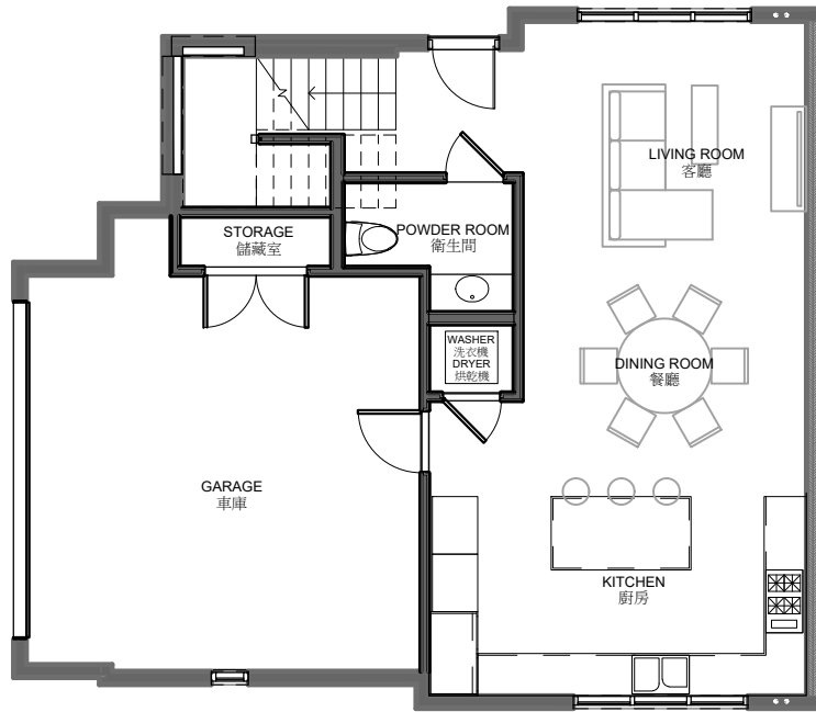
GARAGE 車庫 391 S.F.
