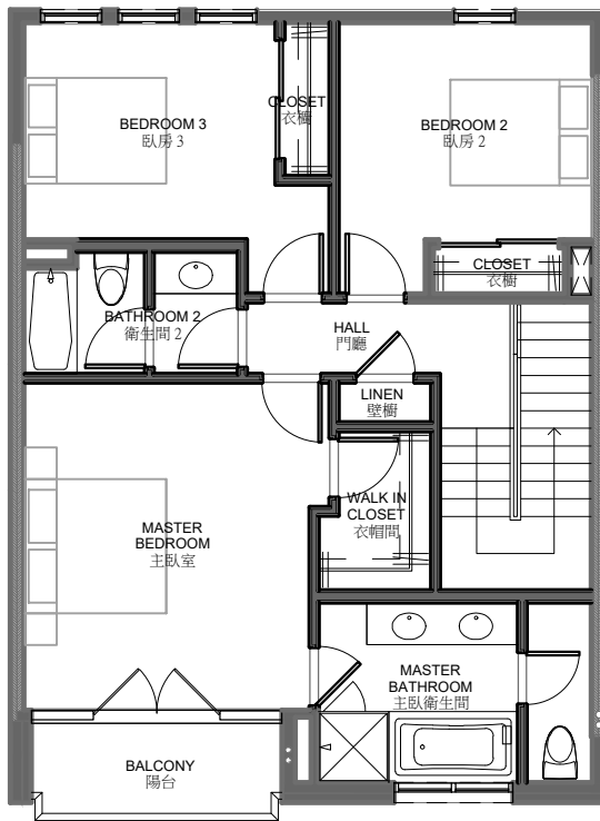
First Floor Plan 1,020 S.F. 一樓平面圖
