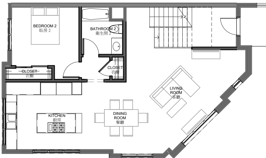
First Floor Plan 1,101 S.F. 一樓平面圖
